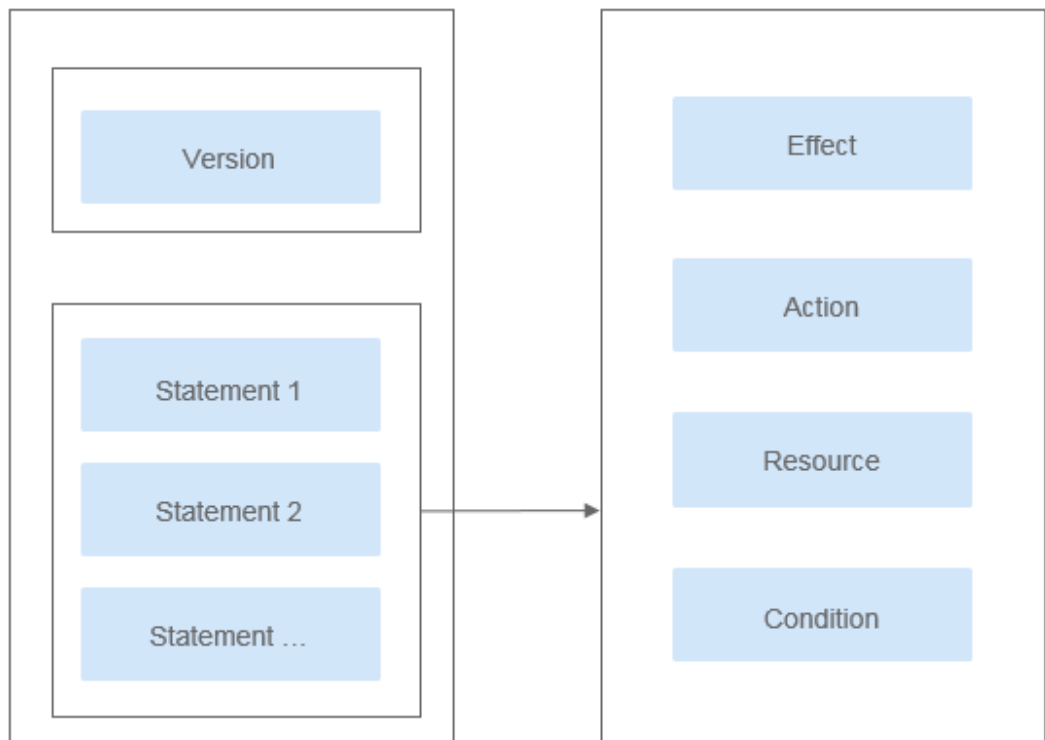
图 2-1 策略结构
