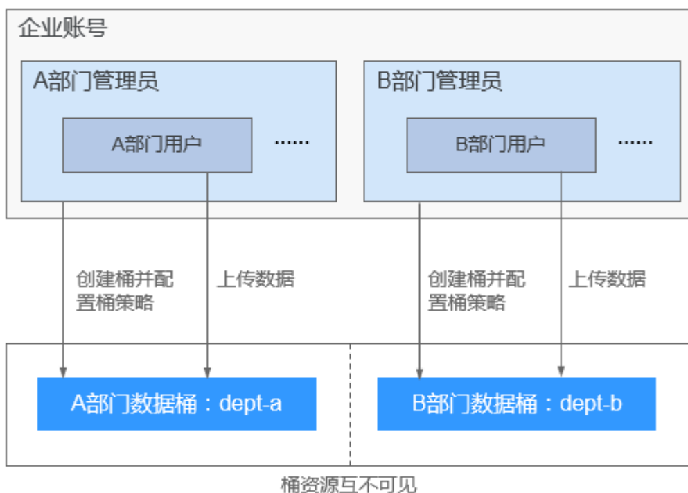
图 5-12 逻辑关系
